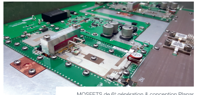
MOSFETS de 6 e génération & conception Planar
