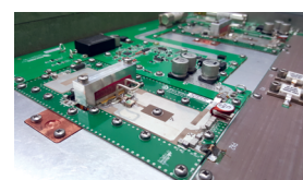
2 paletas RF de diseño planar de 1,25 kW cada una
