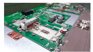
2 paletas RF de diseño planar de 1,25 kW cada una
